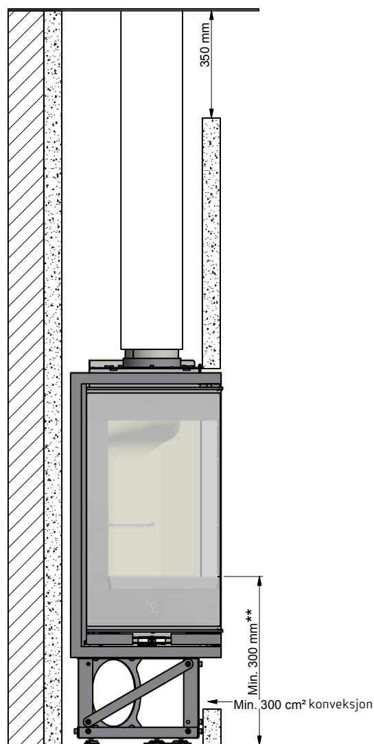
Oppstilling med isolert loddrett røykrør
