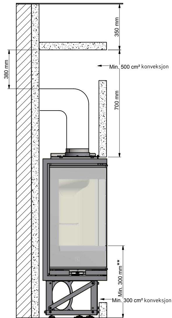
Oppstilling med uisolert kneør
