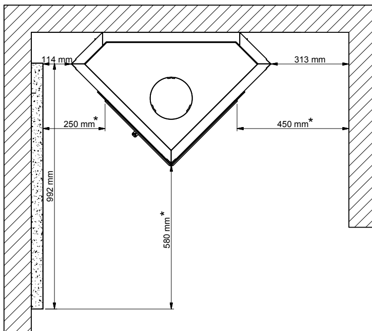
Parallelloppstilling
