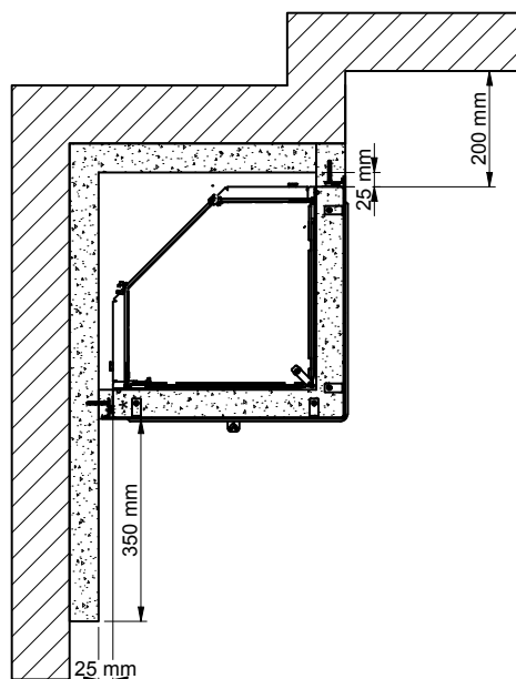
45° hjørneoppstilling
